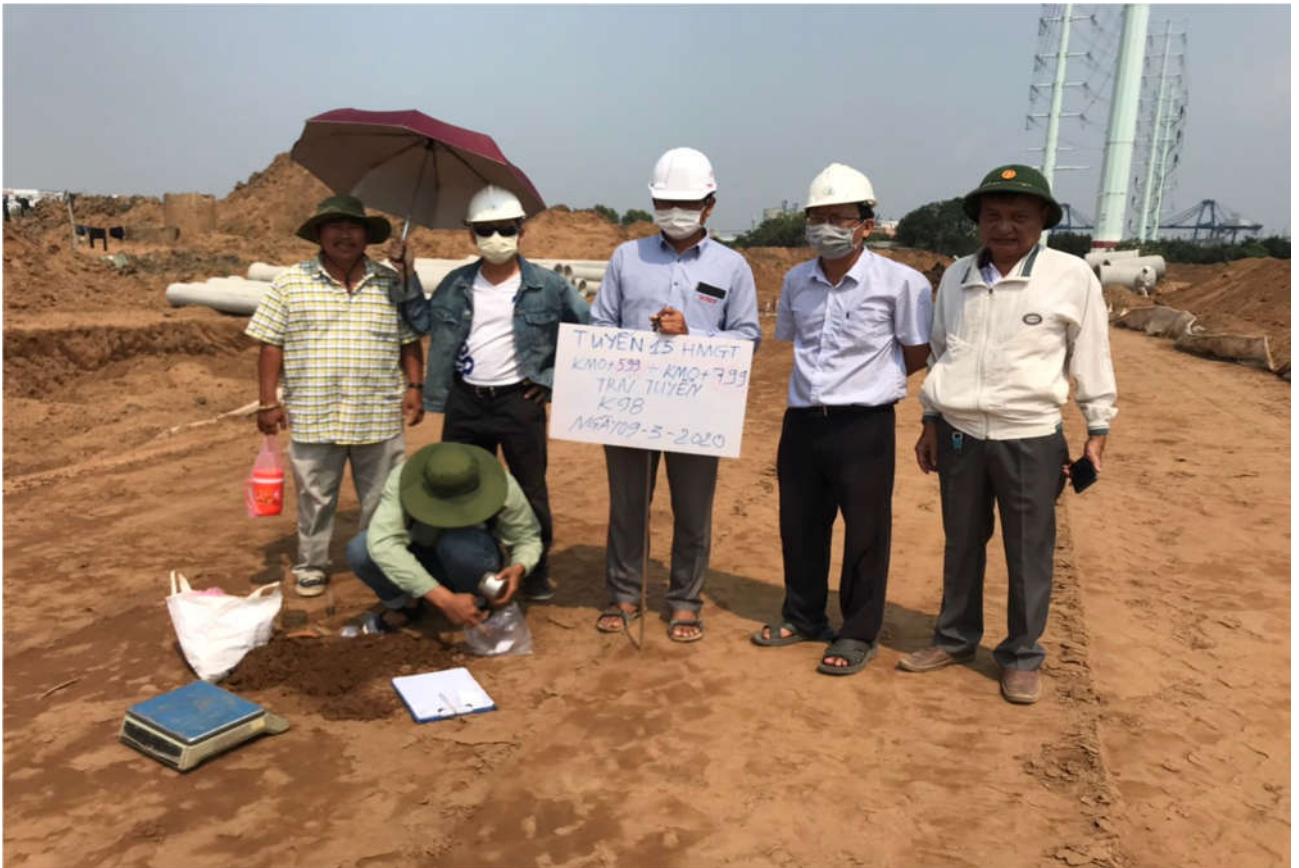
Kiểm tra độ chặt K 98, đường 15
